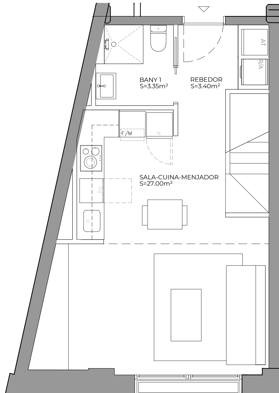
PLANTA INFERIOR
