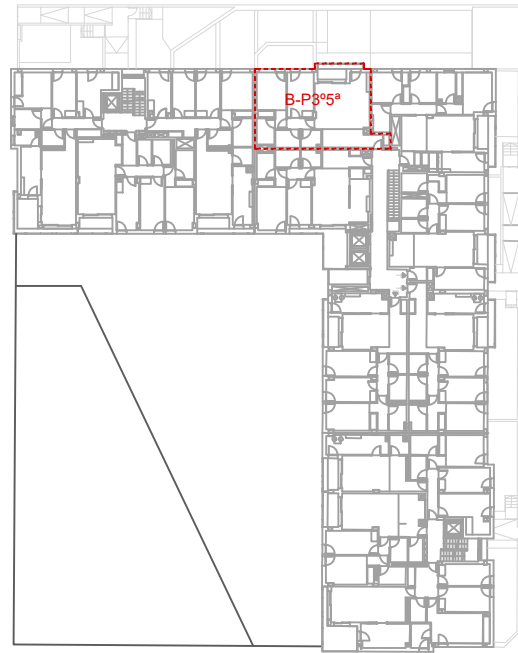
Planta tercera B 3º-5ª (1/2)
