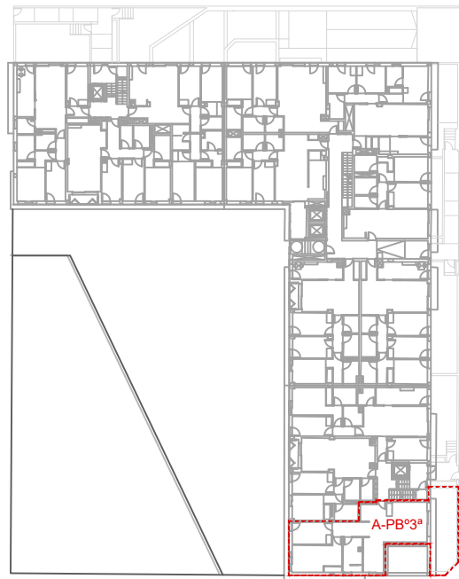
Planta baja A B- 3° (2/2)
