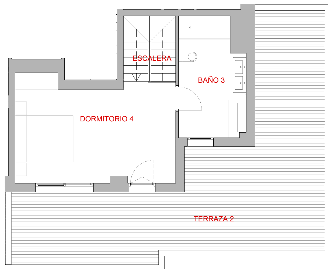
Planta Ático
